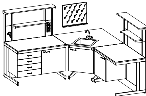
Стол-мойка угловая
