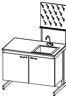
Стол-мойка СЛО-512-22х с сушилкой на кронштейне СЛО-900-04Т
