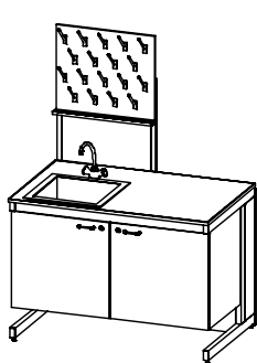
Стол-мойка СЛО-512-12х с сушилкой на кронштейне СЛО-900-03Т
