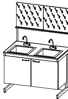
Стол-мойка СЛО-512-32П с сушилкой на кронштейне СЛО-900-05Т
