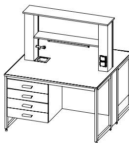
НЛО-32-42-4х с подвесной тумбой НЛО-41-10-х0
