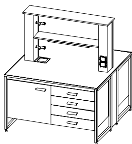
НЛО-32-42-5х с подвесной тумбой НЛО-42-40-х0
