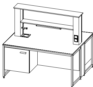
НЛО-33-42-4х с подвесной тумбой НЛО-41-10-х0
