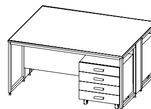
НЛО-33-42-0х с подкатной тумбой НЛО-45-40-х1
